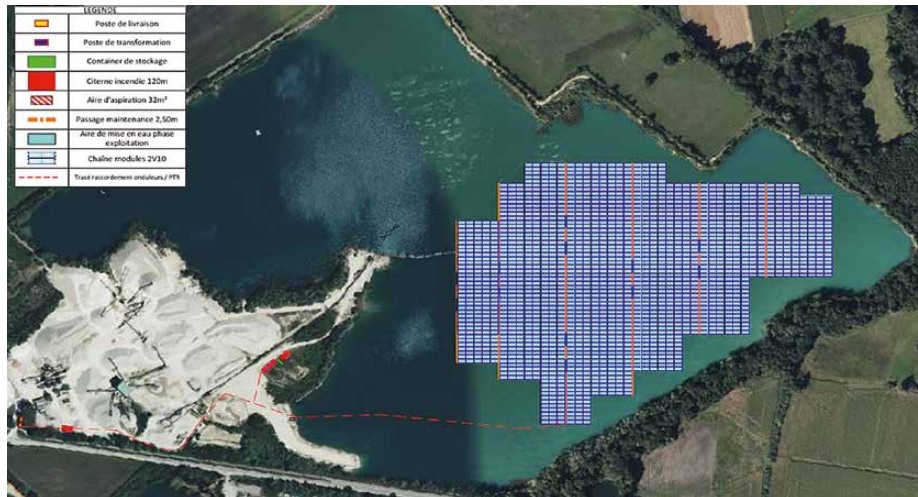
Schéma d'implantation de la centrale photovoltaïque (Extrait du permis de construire)
